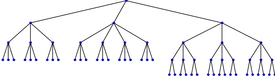
FIG. 6.3. An optimal T^*(39)
