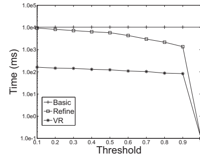
Fig. 14. Gaussian pdf.
